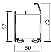
HOL.057.004 THK. 1.4mm - 1.158 Kg/m
