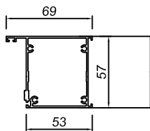
HOL.057.001 THK. 1.4mm - 1.081 Kg/m
