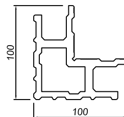
HOL.057.006 THK. 6.0mm - 6.744 Kg/m
