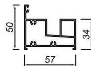
HOL.057.003 THK. 1.4mm - 0.967 Kg/m
