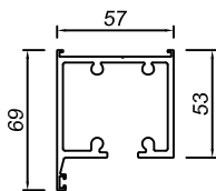
HOL.057.002 THK. 2.9mm - 1.958 Kg/m
